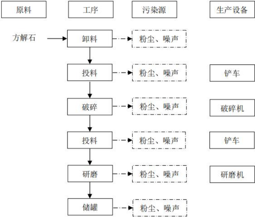
图 2-2 碳酸钙粉生产工艺流程图
